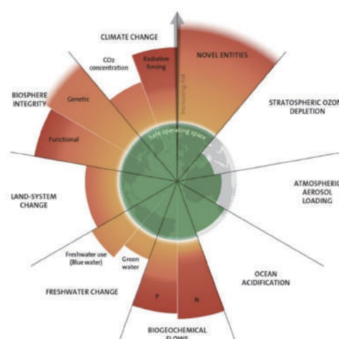
圖25 | 2023 年地球限度系統圖
